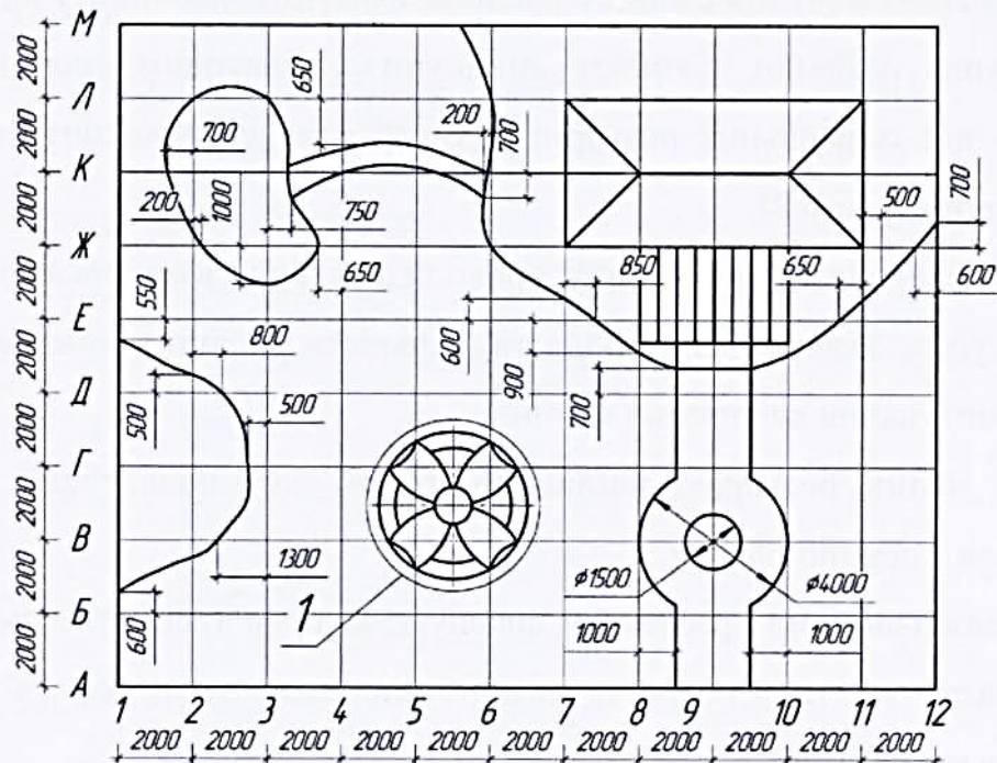
Рис. 6.3. Розбивочний кресленник.
