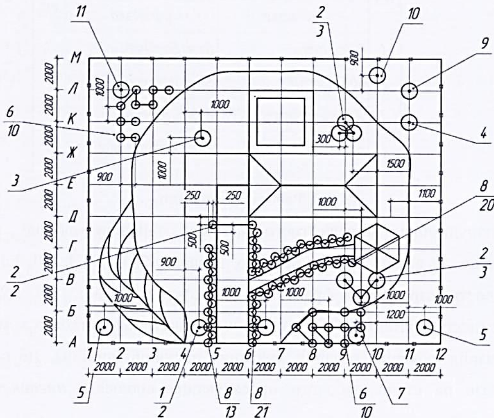
Рис. 6.2. Посадковий кресленник.
