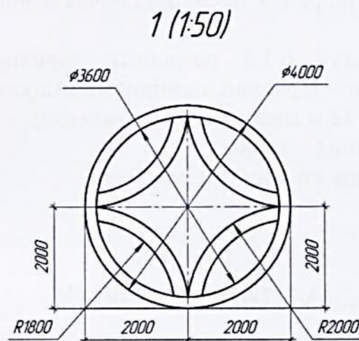
Рис. 6.4.
