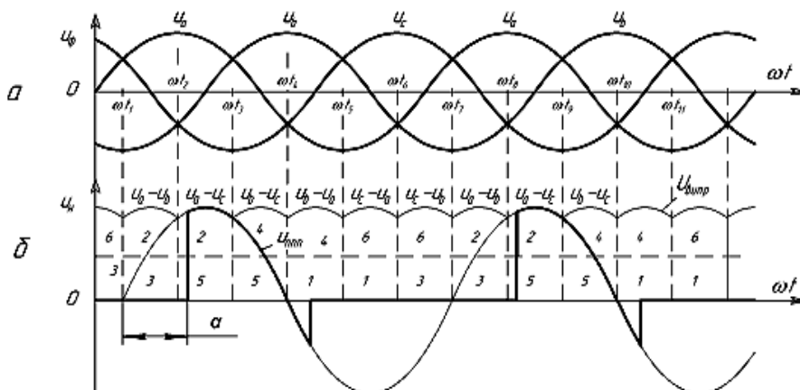
Рисунок 3 – Графіки миттєвих значень напруги мережі живлення (a) і на виході перетворювачів напруги при динамічному гальмуванні (b):
