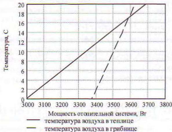
Рис. 2. Зависимость температуры воздуха в грибнице и теплице от мощности отопительной системы
